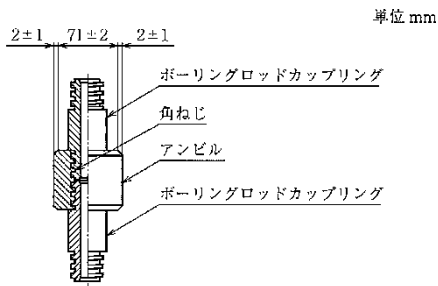
アンビルの標準形状
